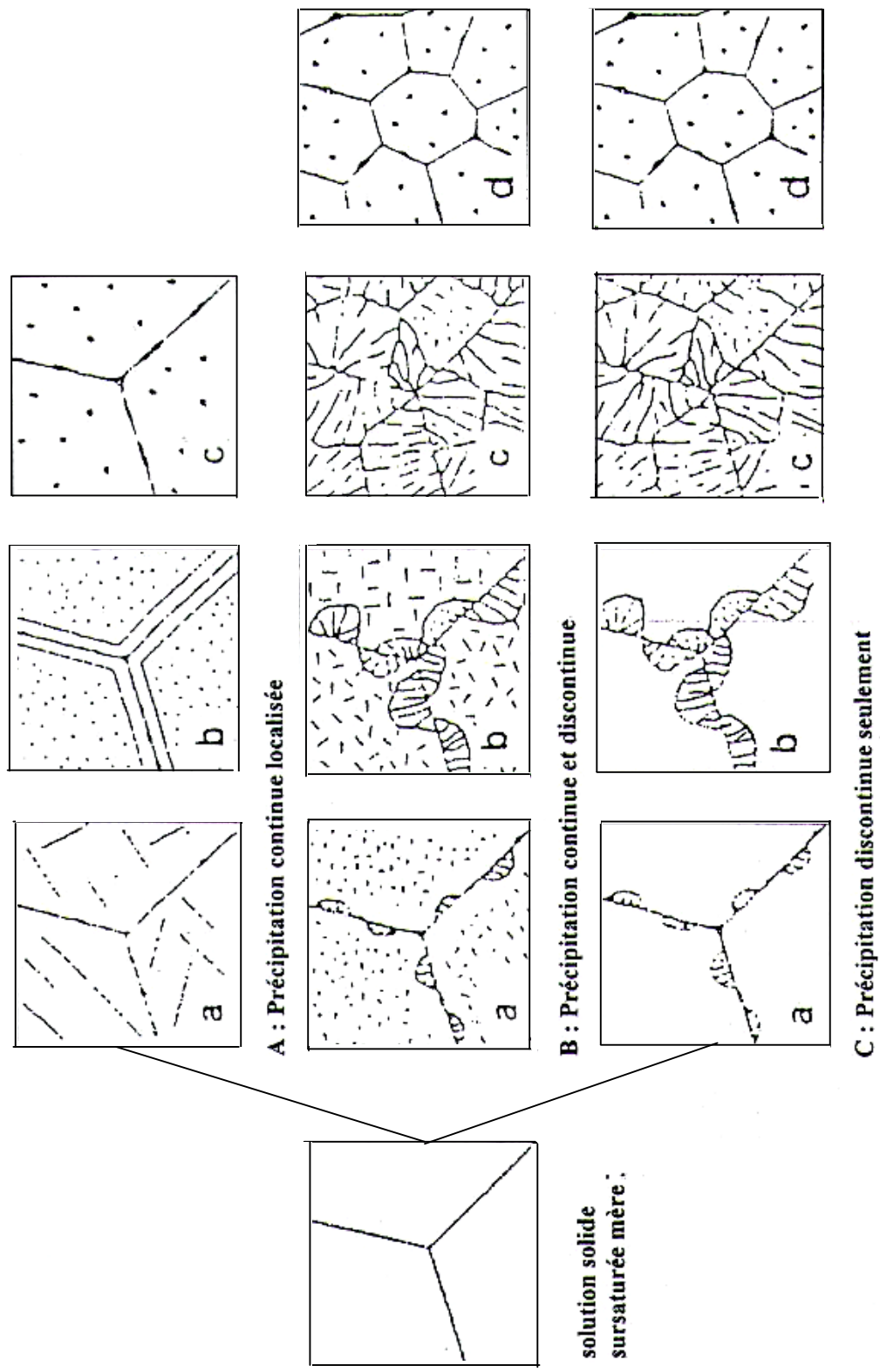
Figure 13. Représentation schématique de la plupart des microstructures et leur caractéristiques, observées par microscope optique durant les divers stades de précipitation à partir de la solution solide sursaturée [40].
