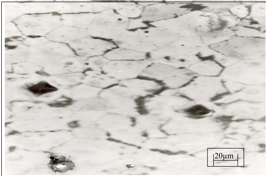
Figure 76. Double couture ou « Mécanismes S » dans l'alliage Al-30 mass.%Zn déformé de 48%, homogénéisé pendant 21 jours à 450^{\circ}\text{C} , trempé dans la glace, ensuite vieilli à 160^{\circ}\text{C} pendant 22 heures
